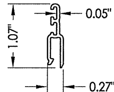
19 SILL RISER
